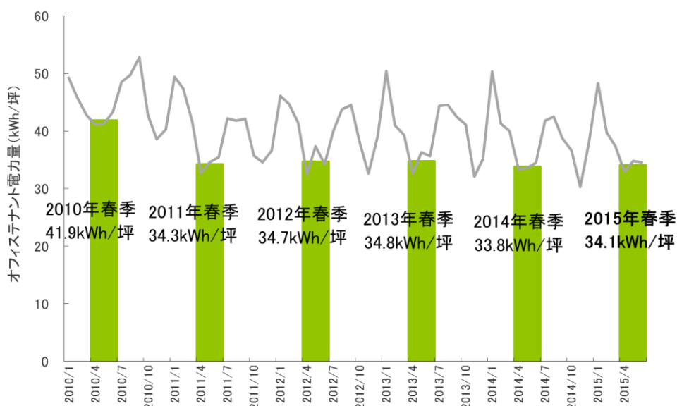
図表 2 オフィステナント電力量春季平均（4～6月、東京電力管内）の推移
